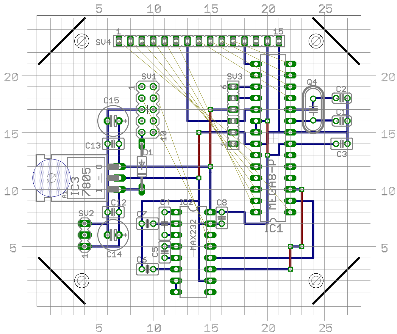
Wandbedienung - MC und Interface wall-control - mc and interface
